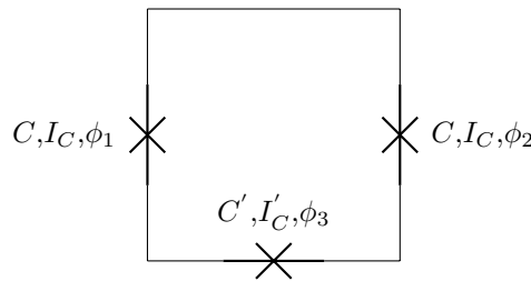
Abbildung 1: Flussqubit aus drei Josephson-Kontakten
